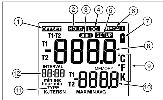
Kuva 2. Näytön osat
